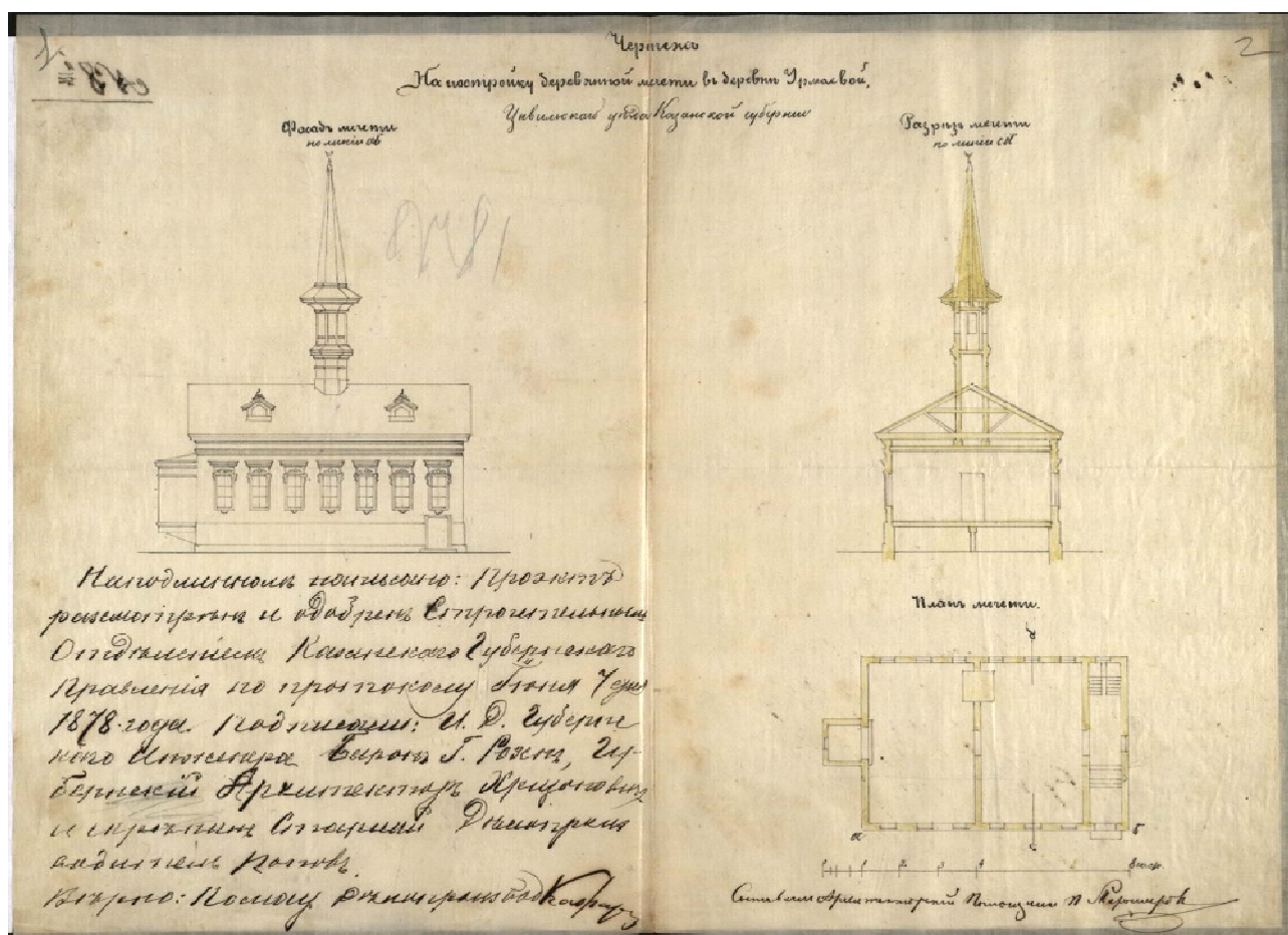
Урмай авылы агач мәчете планы. 1878 ел. ТР ДА. 2 ф. 14 тасв. 616 эш.
